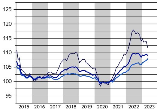
Indexverlauf (Gesamtindizes)
