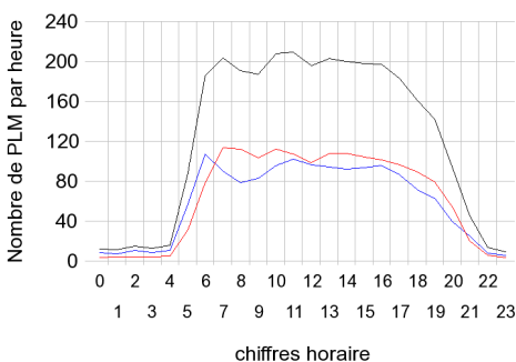
Trafic journalier moyen des jours ouvrables
