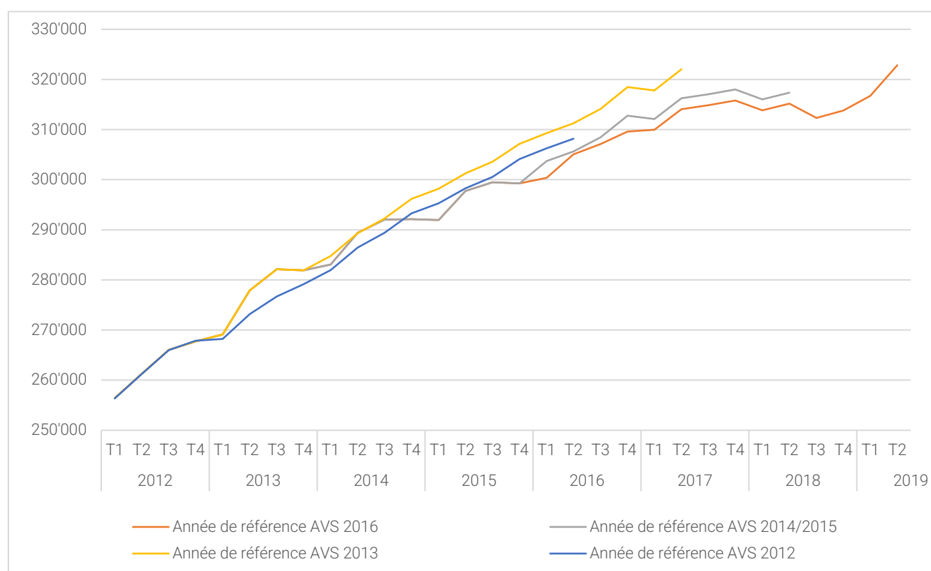
Figure 2: Nombre de frontaliers de nationalité étrangère, par année de référence AVS, 2012 à 2019
