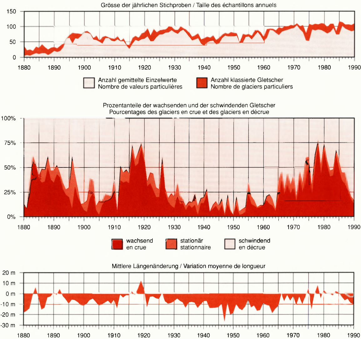
G2.1 Lageänderung der Gletscherenden in den Schweizer Alpen 1880 - 1990 Variation des fronts glaciaires dans les Alpes suisses de 1880 à 1990
