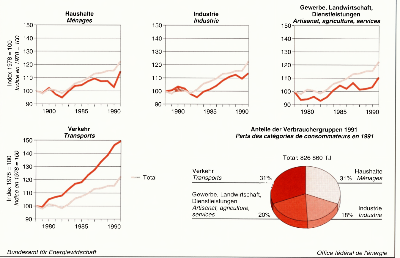
G8.5 Endenergieverbrauch nach Verbrauchergruppen Consommation finale d'énergie par catégorie de consommateurs
